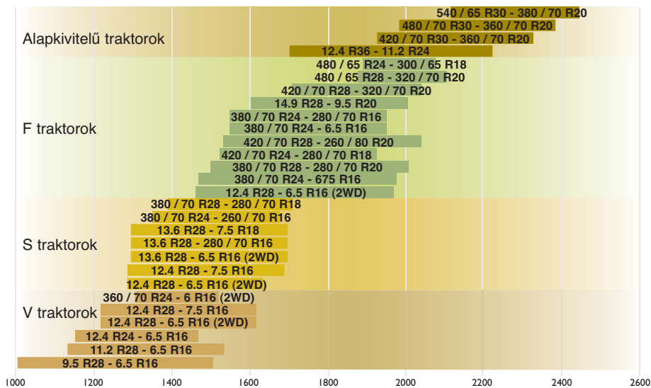
A traktorok minimális-maximális szélessége (mm) a hátsó kerék méretétől függően
